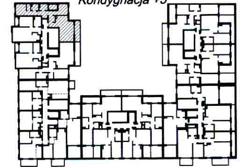
Rzut 4 piętra Kondygnacja +5
